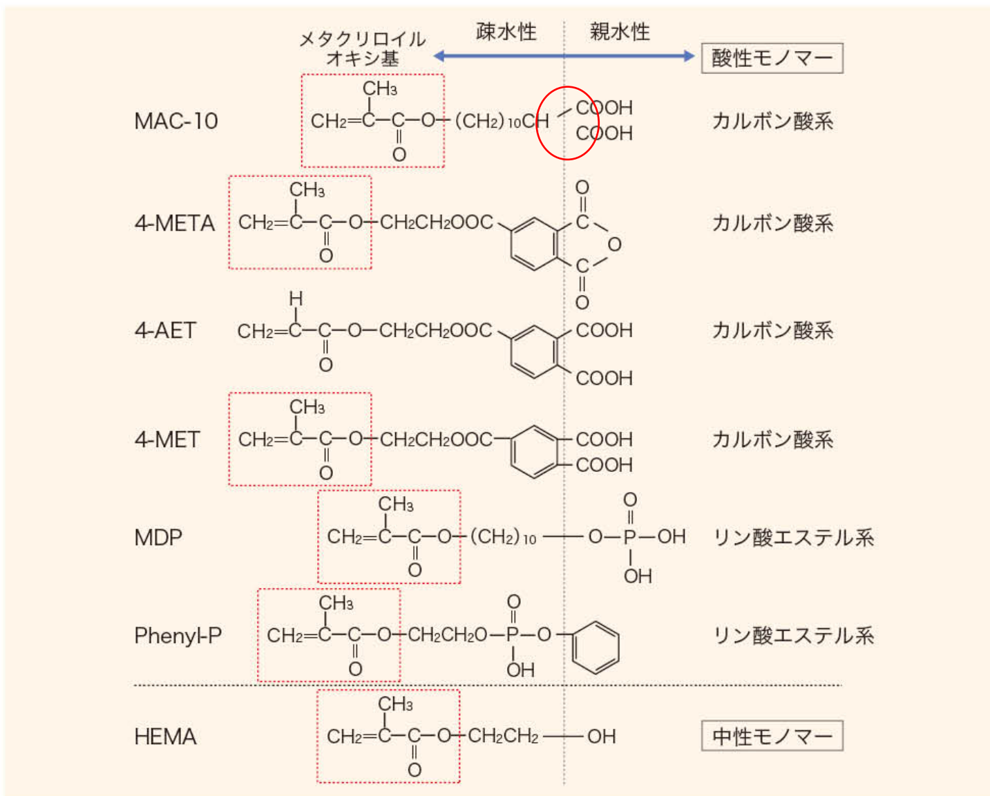
■ 図 5-15 ■ 代表的な機能性モノマーの構造
