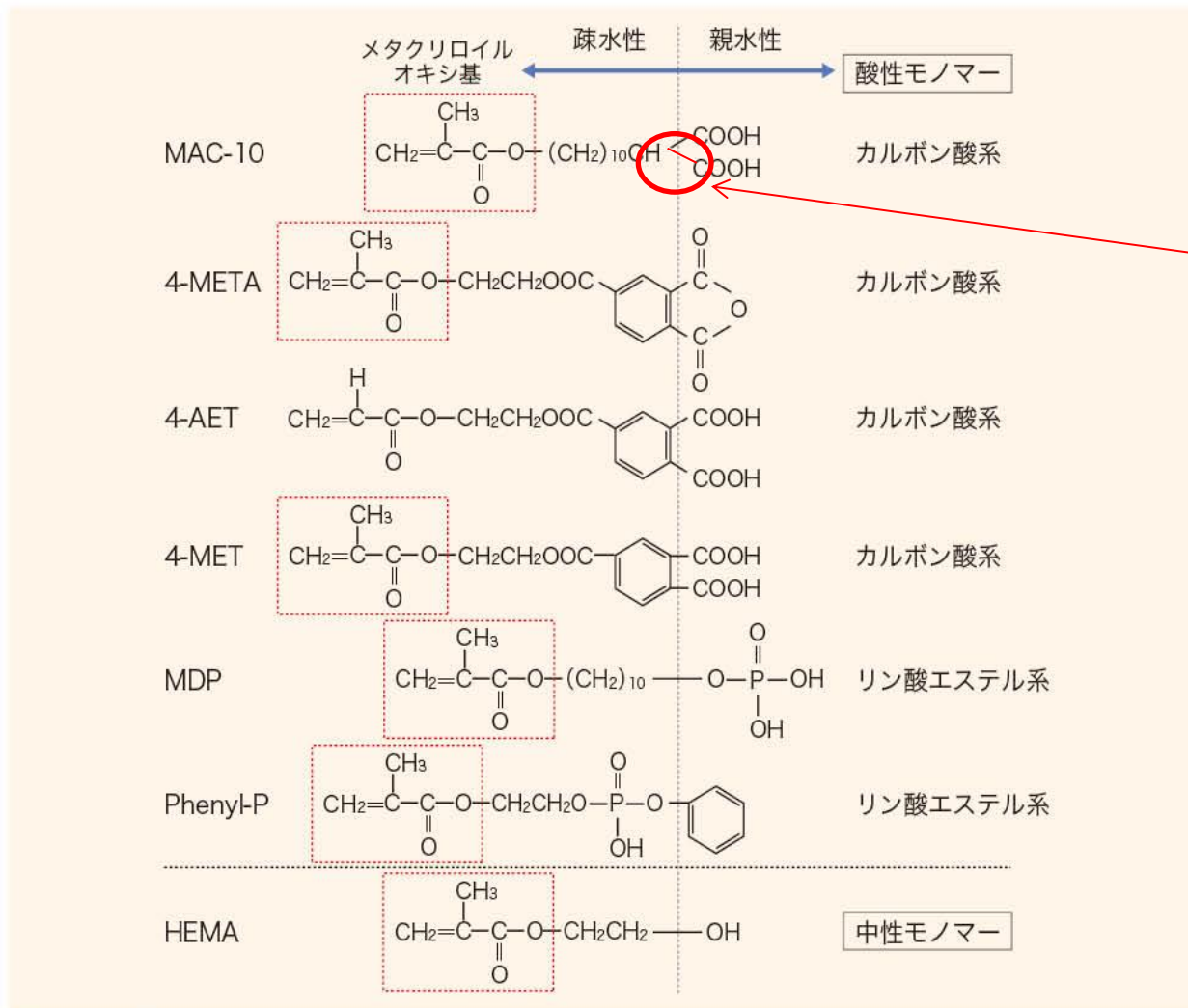
■ 図 5-15 ■ 代表的な機能性モノマーの構造 (長谷川二郎 ほか編：現代歯科理工学, p.116, 大野弘機：医歯薬出版, 1996 より)
