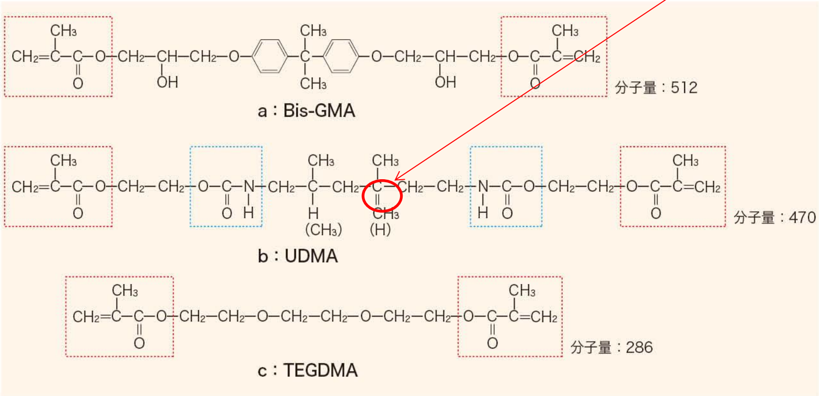
■ 図 5-3 ■ コンポジットレジンに使用される代表的なモノマーの構造
